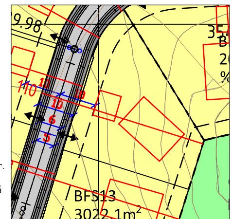
Kartutsnitt MstK = 1:1000
